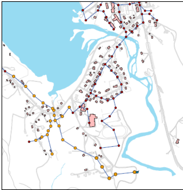
Fig 14 Oversiktskart vannforsyning (fra kommunen).
